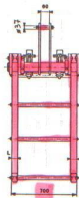
Simplex Profil 62x40: L = 40 Profil 70x49: L = 50
