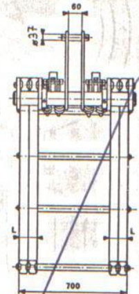
Duplex Profil 62x40: L = 80 Profil 70x49: L = 100
